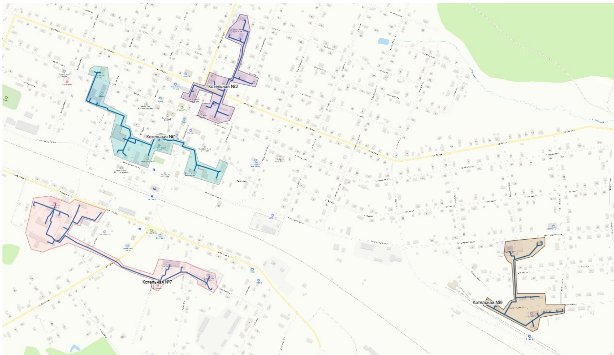
Рисунок 3 – Зоны действия источников централизованного теплоснабжения
